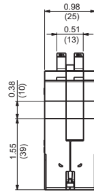
HOMT Tandem
